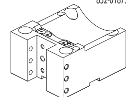
KMS-T00186 (25x25 mm) KMS-T00187 (20x20 mm)
